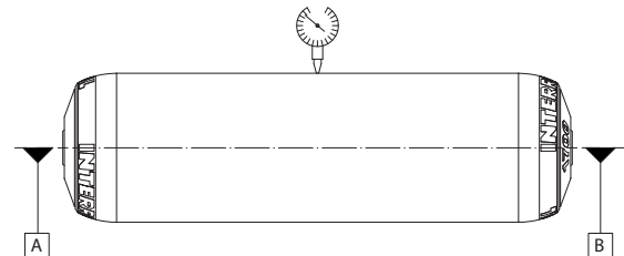
Fig.: Medición de la desviación de concentricidad
