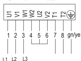
Y 3-Ph-Motor
