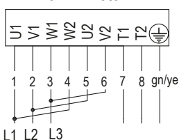
△ 3-Ph-Motor
